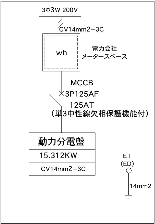
動力引込開閉器 結線図
