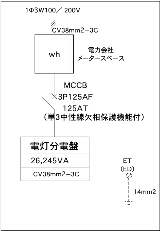
電灯引込開閉器 結線図
