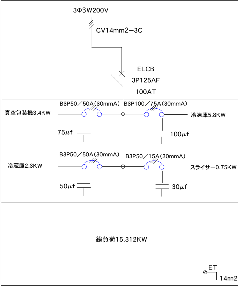
動力分電盤 結線図
